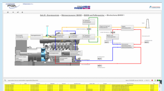
webbasiertes SCADA-System Energiezentrale, Wärme'erzeugung / BHKW und Pufferspeicher
